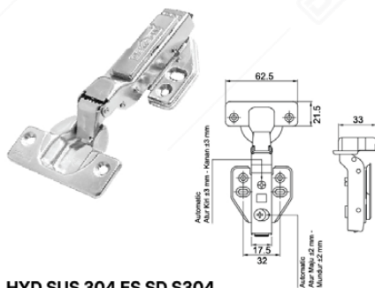
HYD SUS 304 ES SD S304 HALF OVERLAY PSS
