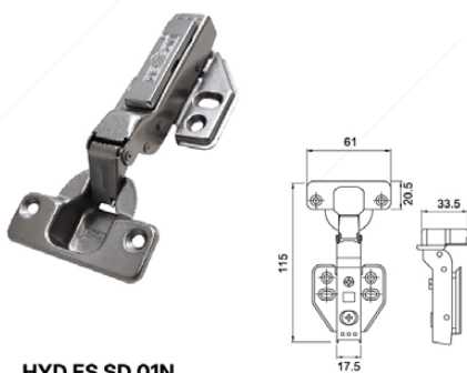
HYD ES SD 01N HALF OVERLAY TN
