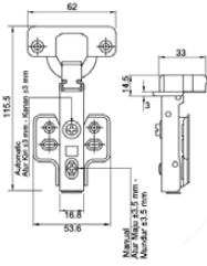
HYD ES SD 03 FULL OVERLAY SN
