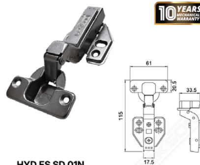
HYD ES SD 01N INSET TN
