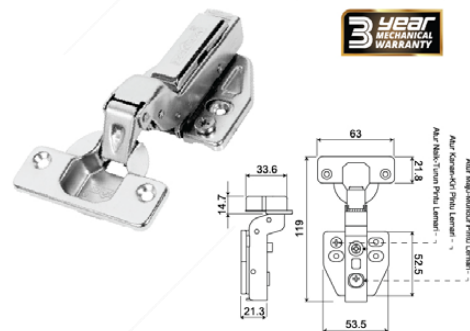
HYD ES SD D8383 3D ADJ INSET SN
