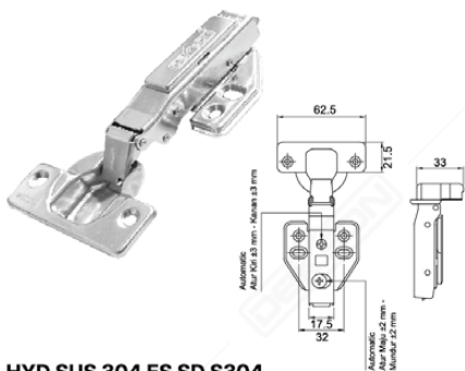
HYD SUS 304 ES SD S304 FULL OVERLAY PSS
