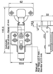
HYD ES SD 03 HALF OVERLAY SN
